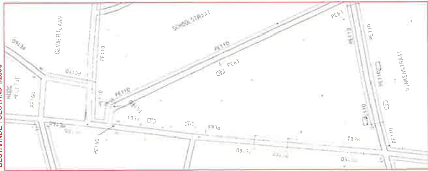
BESTAANDE TOESTAND 1/2500
