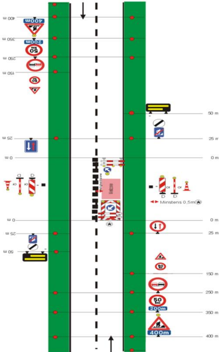
Bijlage 2: Signalisatieschema t.p.v. werkzone.
